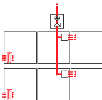
- installation d'extraction d'air avec prises d'air neuf
