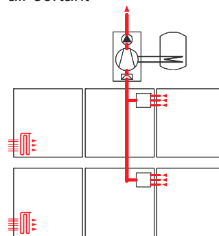
- aération douce avec pompe à chaleur à air sortant
