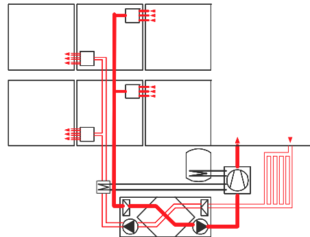
- aération douce avec pompe à chaleur à air sortant
