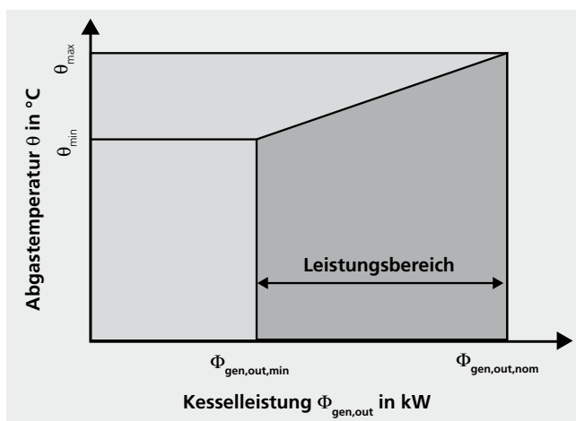
Abgastemperaturdiagramm
