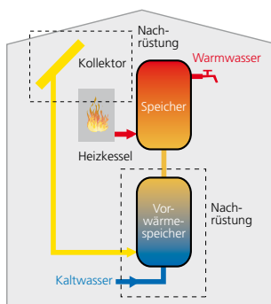
System A: System mit Vorwärmespeicher
