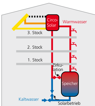
System E: CircoSolar-Anlage
