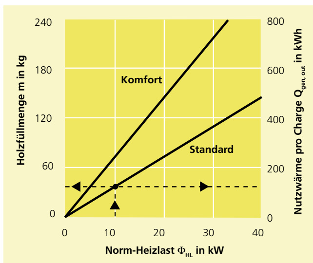
Auslegung Stückholz-kessel
