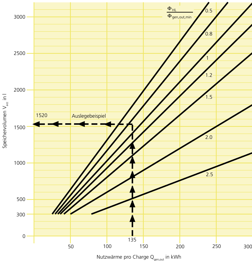
Speicherdimensionierung
