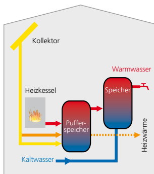
System C: Mehrspeichersystem mit Pufferspeicher
