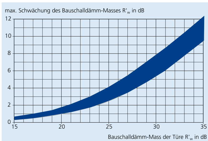
Reduktion des Schalldämmmasses einer Tür durch einen 5 mm bis 10 mm hohen Luftspalt.
