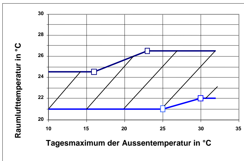
Bild 4: Bereich der Raumlufthtemperatur nach Tagesmaximum der Aussentemperatur
